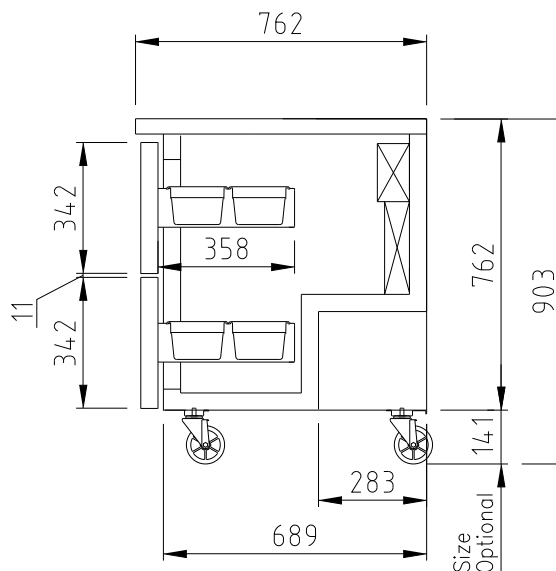
ВИД СБОКУ
