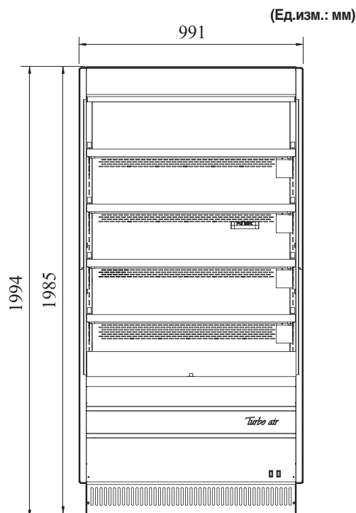
ВИД СПЕРЕДИ
