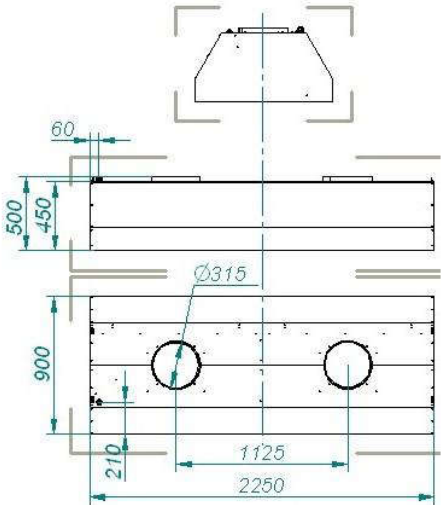
Рис. 3а Зонт вентиляционный ос. тробной ЗВЗ-900-40
