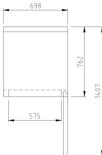
ВИД СВЕРХУ
