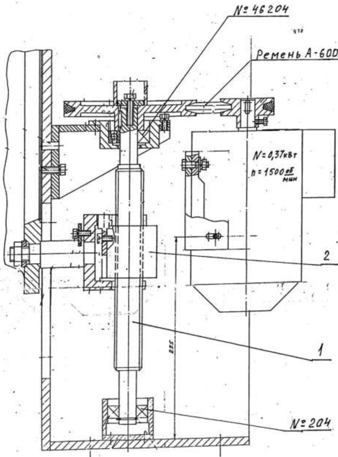
Рисунок 5 Механизм подъема дежи 1. Винт; 2. Гайка.
