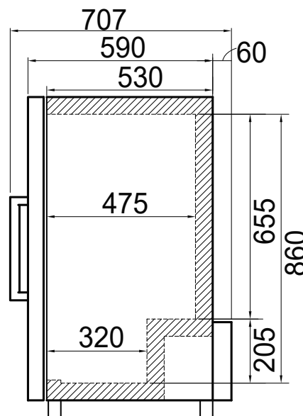
ВИД СБОКУ
