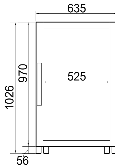
ВИД СПЕРЕДИ
