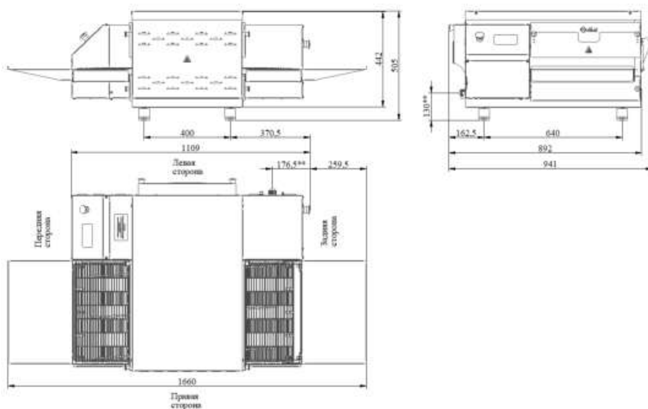
Рис. 1 - Общий вид печи, где ** - подвод электропитания
