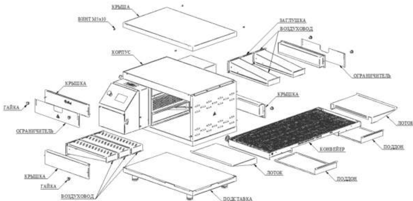
Рис. 4 - Состав изделия
