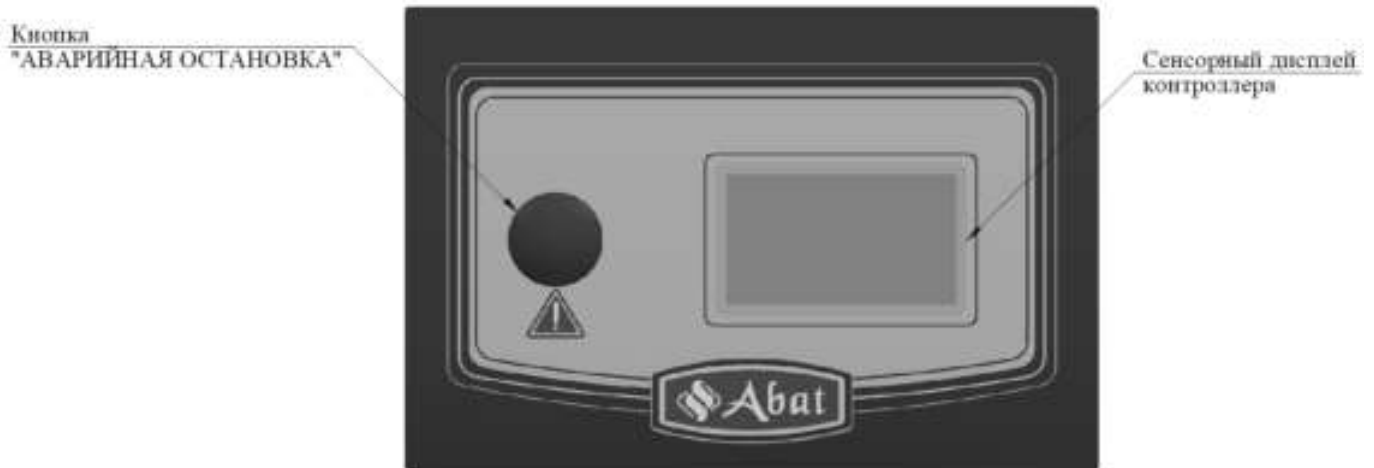
Рис. 5 - Панель управления
