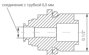
переходник 1/2" x 1/4"
