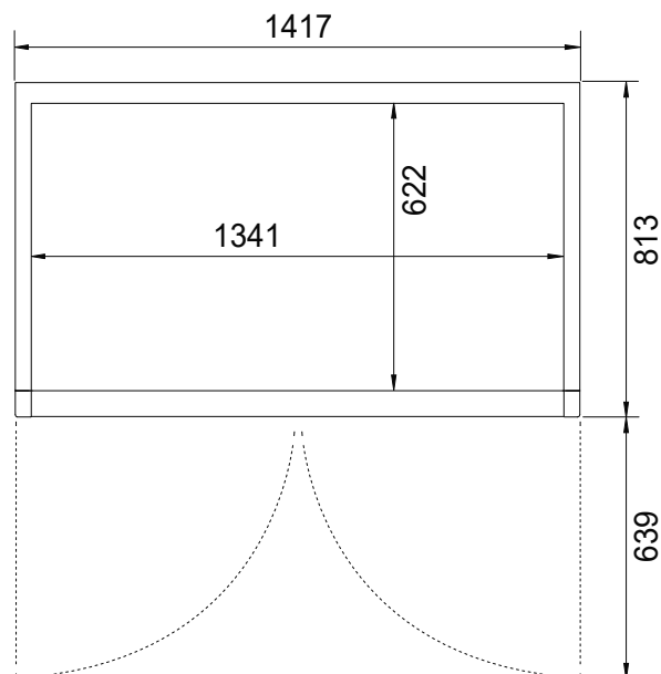
ВИД СВЕРХУ
