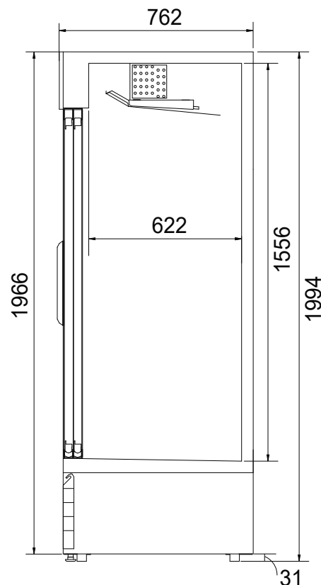
ВИД СБОКУ
