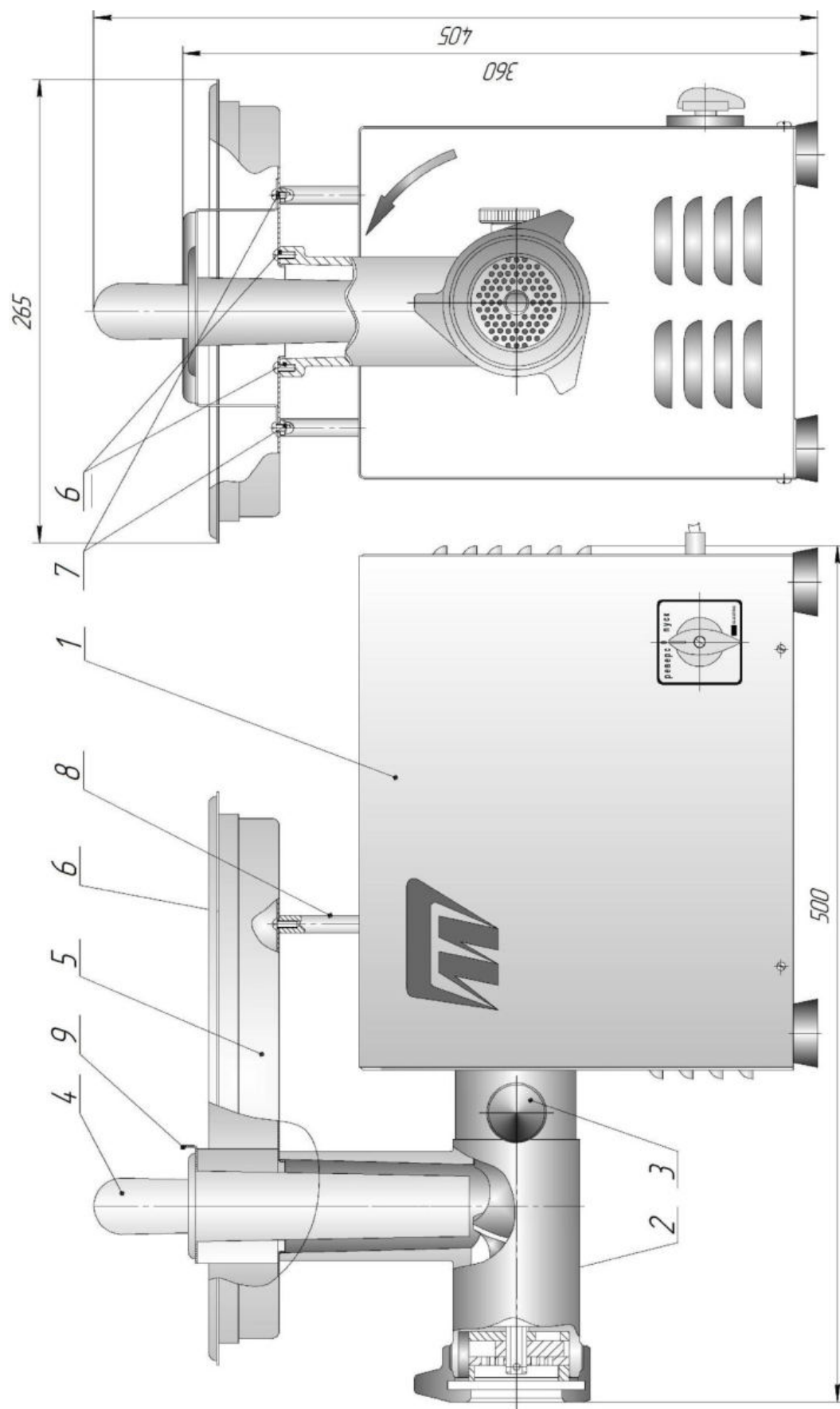
Рисунок – 1 Мясорубка
