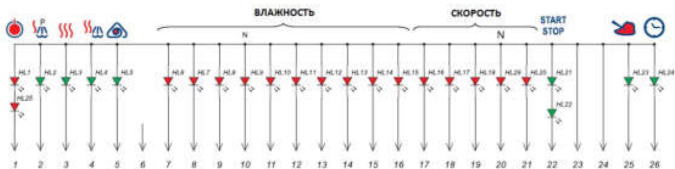
Схема электрическая соединения светодиодов
