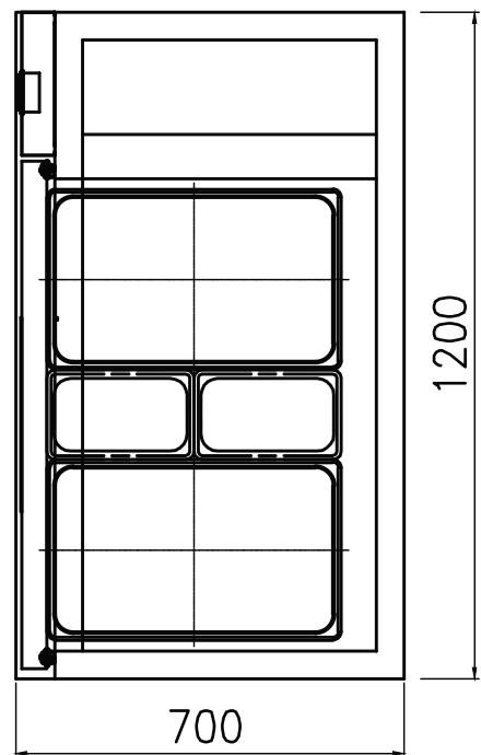
ВИД СВЕРХУ
