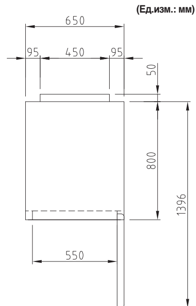
ВИД СВЕРХУ
