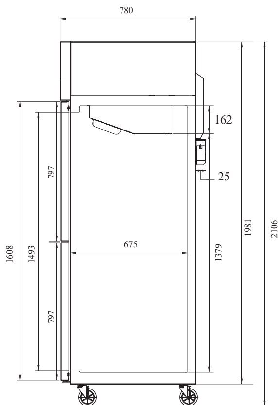
ВИД СБОКУ
