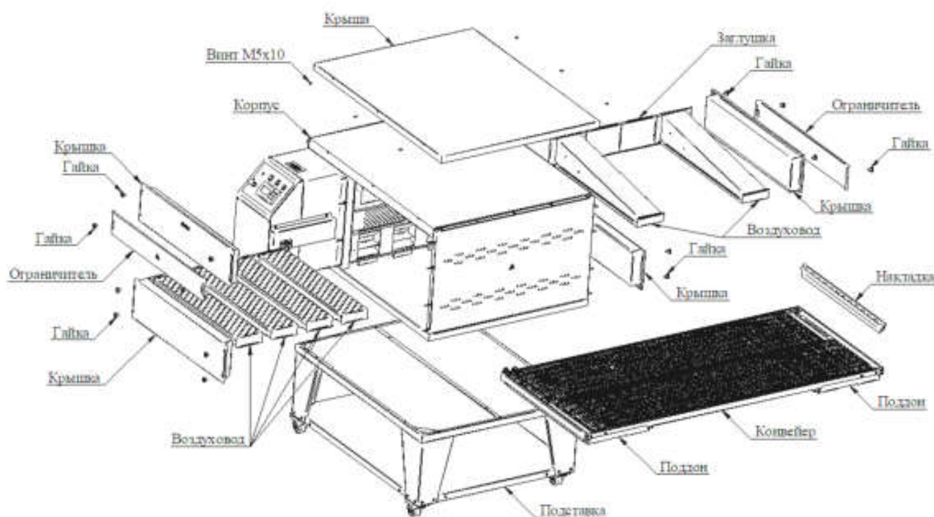
Рис. 3 - Состав изделия
