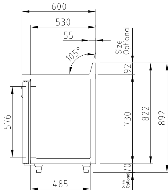
ВИД СБОКУ
