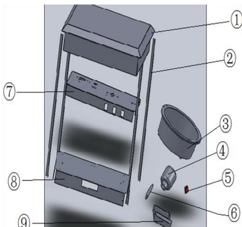
Рис.1 – Аппарат для приготовления попкорна серии VBG
