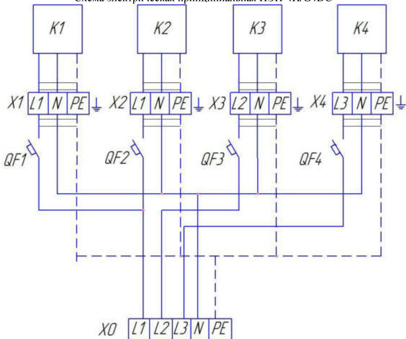
Схема электрическая принципиальная ПЭИ-4Н/G4DC
