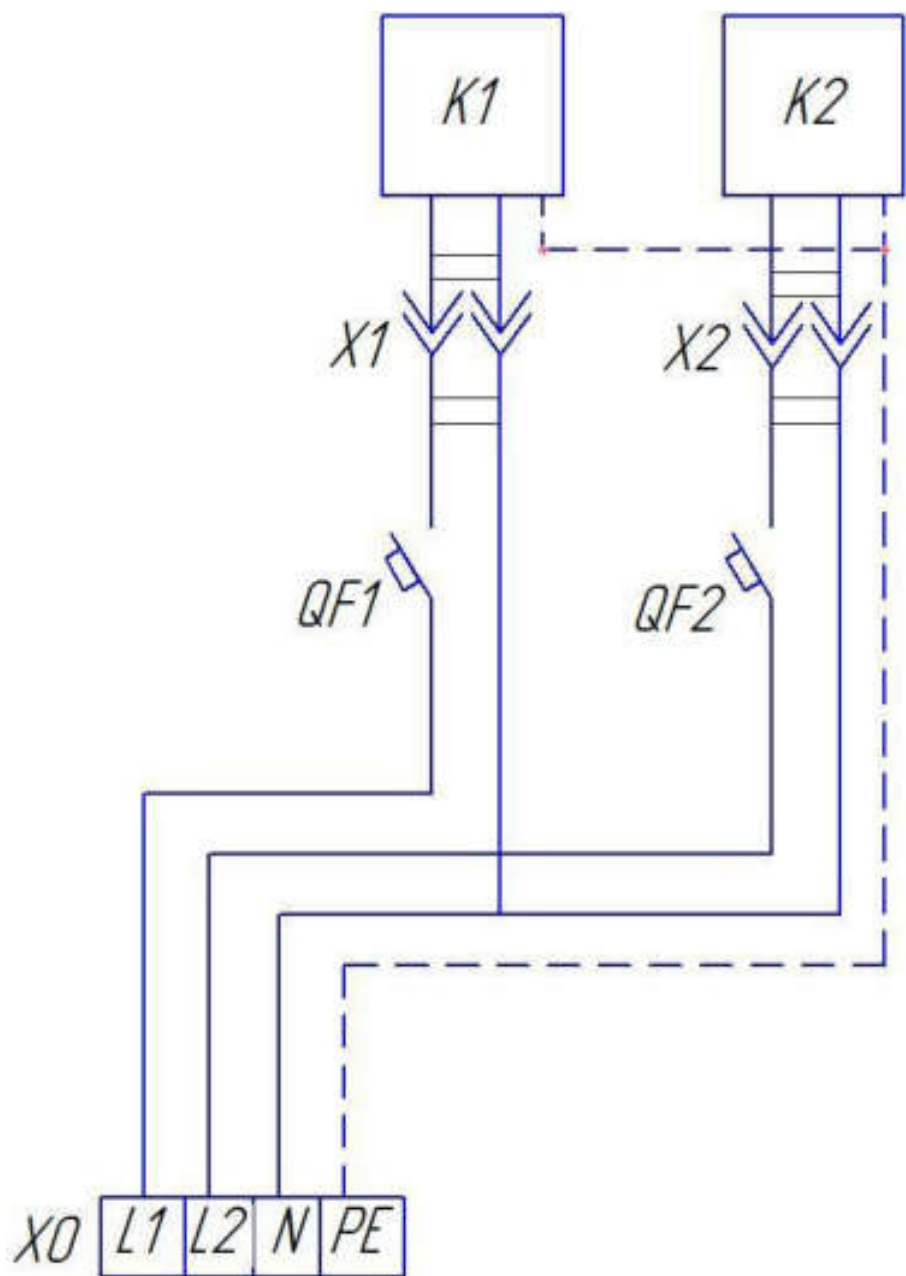
Схема электрическая принципиальная ПЭИ-2HDC
