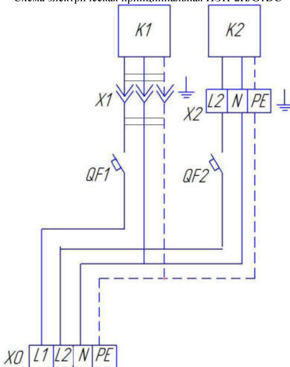
Схема электрическая принципиальная ПЭИ-2Н/G1DC
