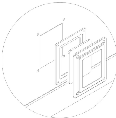
Рис.5 Замена лампы освещения ПР-4М-Э, ПР-05МЭ
