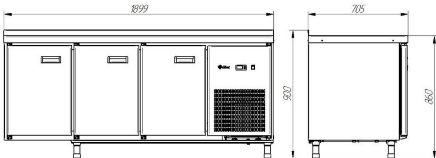
Рис.6. Габаритные размеры СХС-70-02-СО столешница с бортом (дверь, дверь, дверь)*
