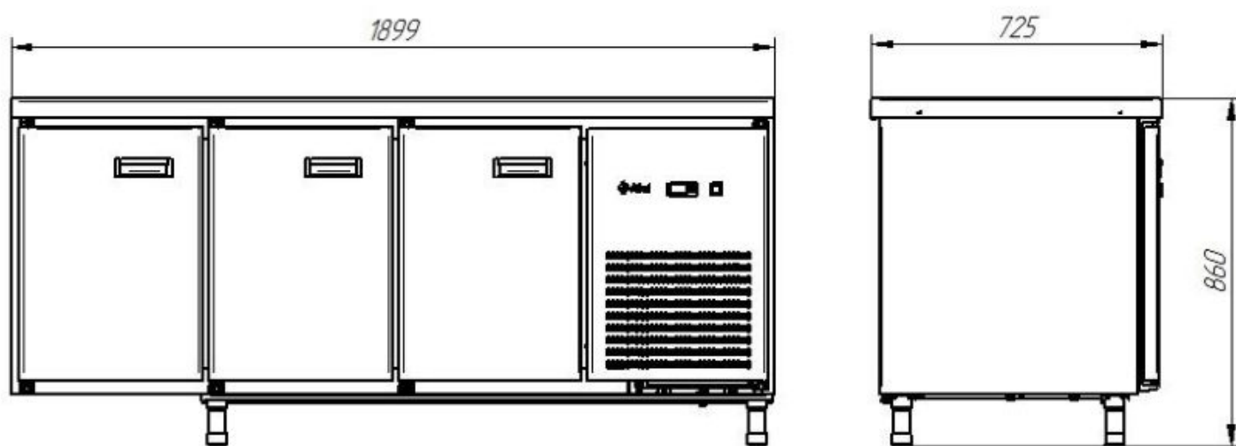
Рис.7. Габаритные размеры СХС-70-02-СО столешница без борта (дверь, дверь, дверь)*
