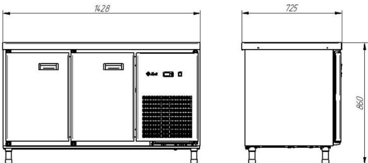
Рис.5. Габаритные размеры CXС-70-01-CO столешница без борта (дверь, дверь)*
