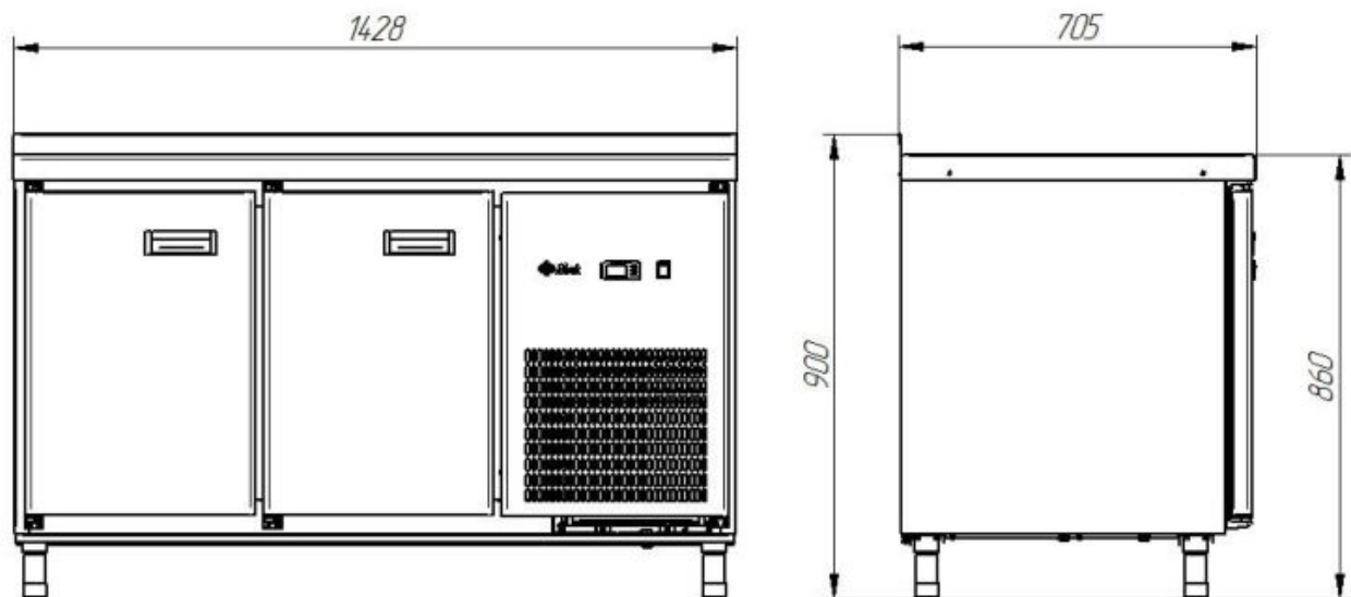
Рис.4. Габаритные размеры CXС-70-01-CO столешница с бортом (дверь, дверь)*
