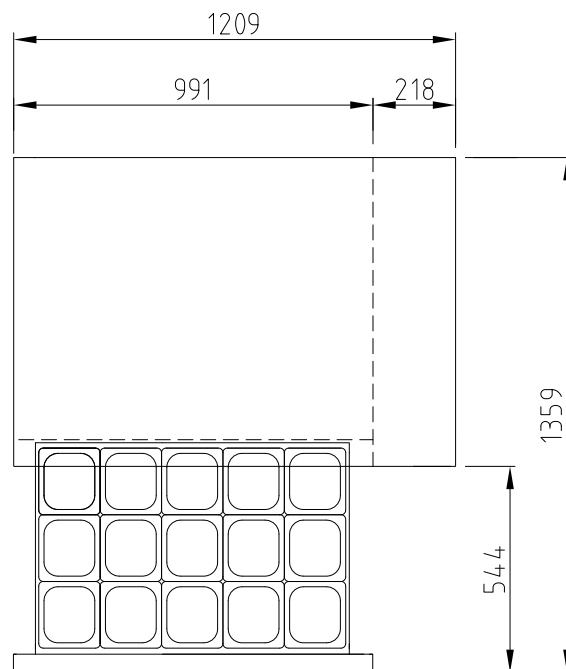
ВИД СВЕРХУ
