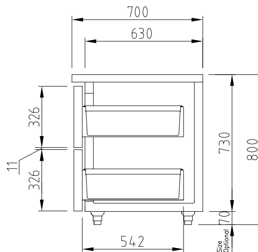
ВИД СБОКУ
