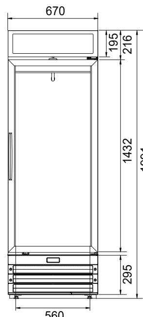
ВИД СПЕРЕДИ
