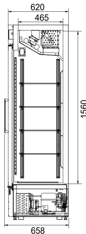
ВИД СБОКУ
