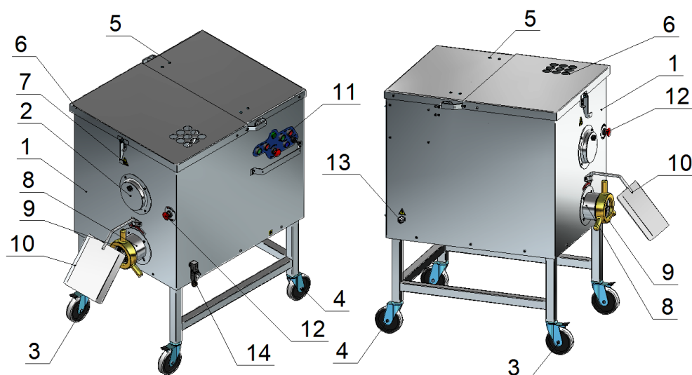
Рис. 1 Устройство мясорубки
