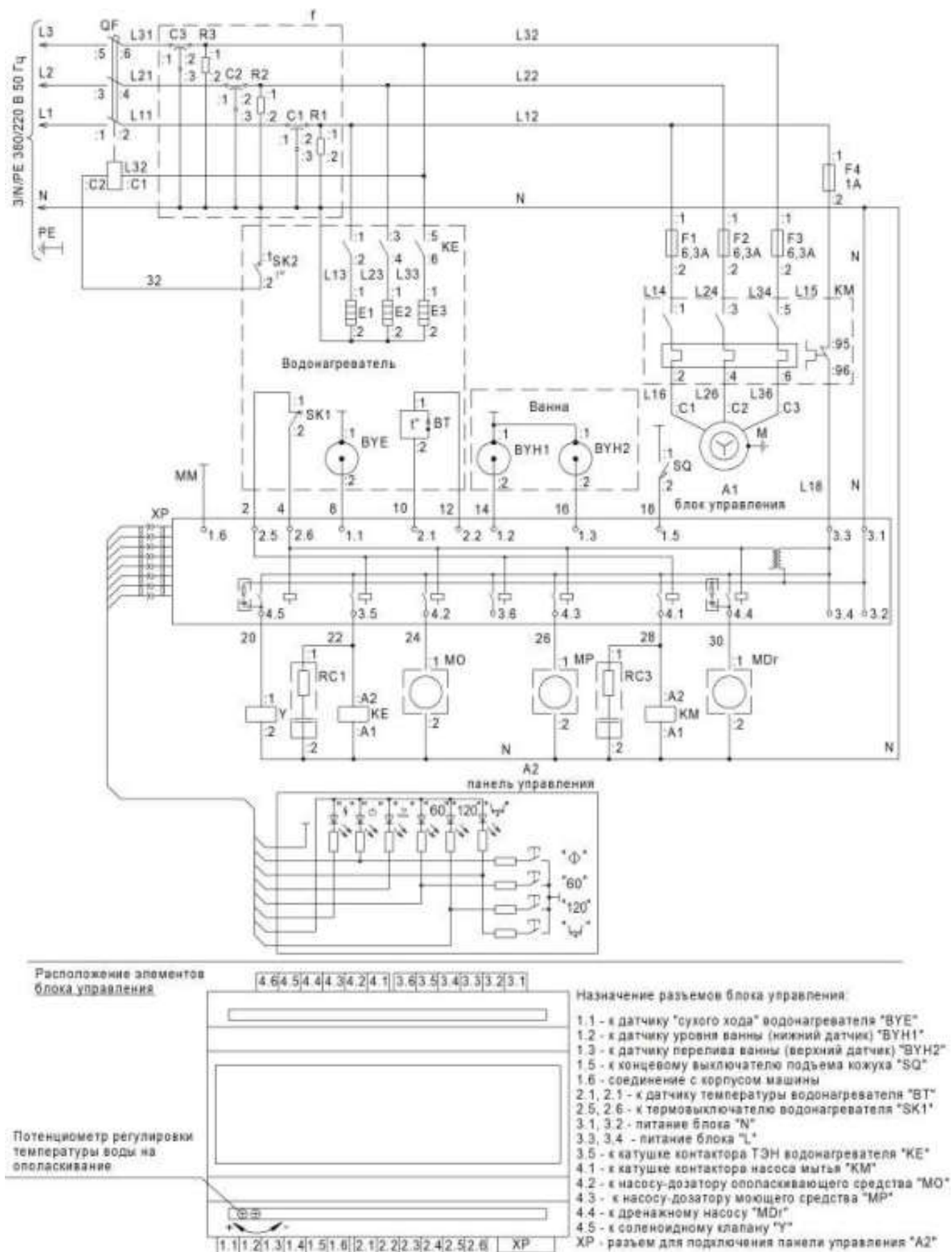
Рисунок 3 – Схема электрическая принципиальная
