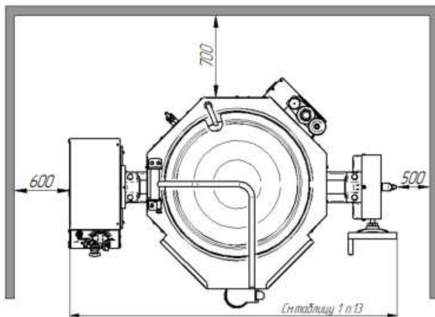
Рис. 4. Установка котла
