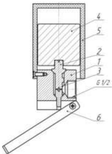
Клапан предохранительный типа КПК ДКАБ.305365.001
