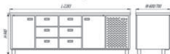
СШС-6,2-2300/ СШН-6,2-2300
