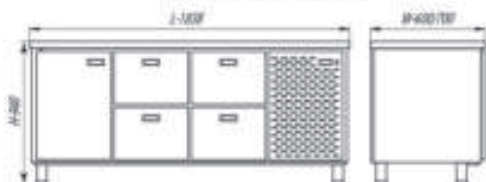
CWC-4,1-1850 / CWH-4,1-1850
