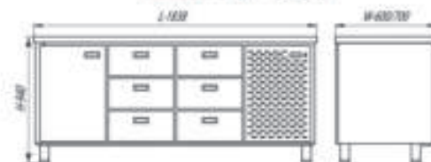
CWC-6,1-1850 / CWH-6,1-1850
