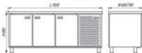
CWC-0,3-1850 / CWH-0,3-1850
