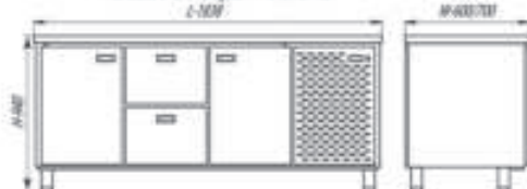
CWC-2,2-1850 / CWH-2,2-1850
