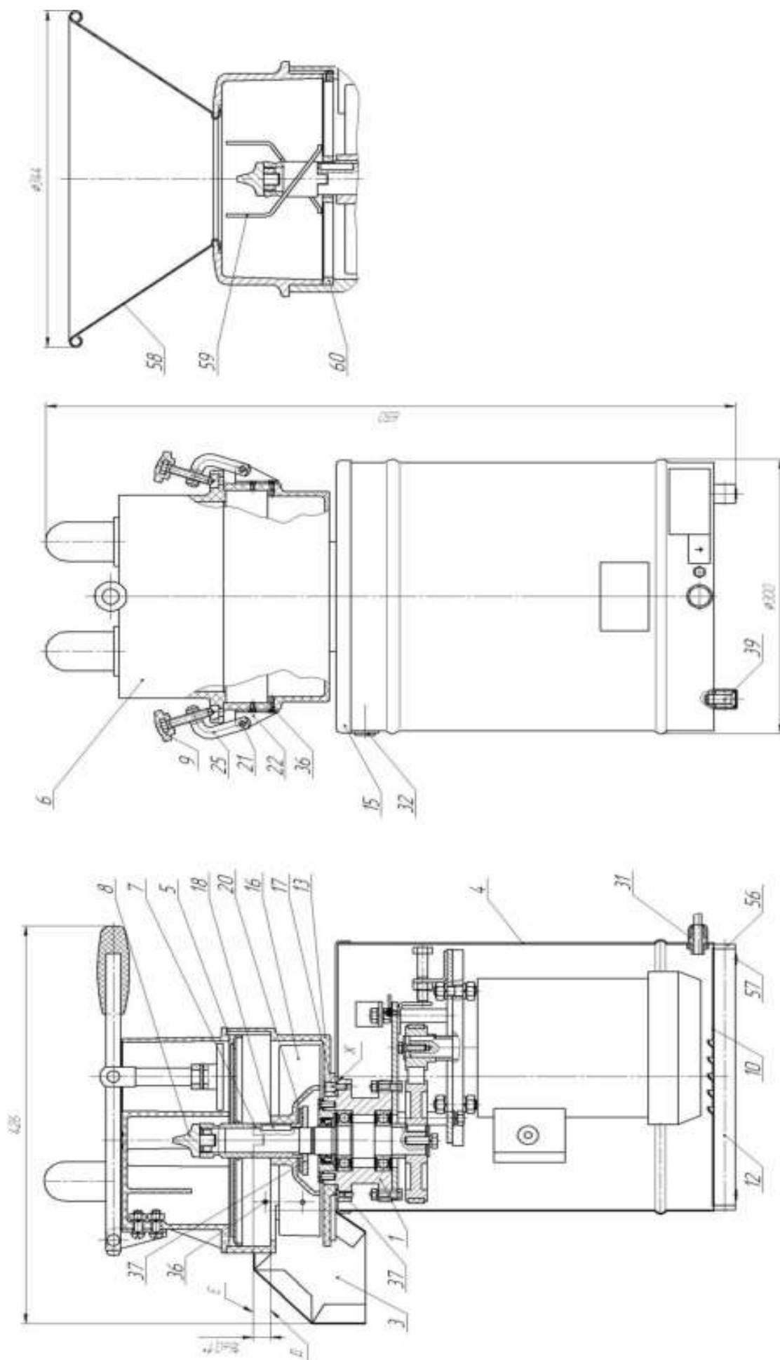
Рисунок 2 Машина обшаривательно-протирочная ОМ-350
