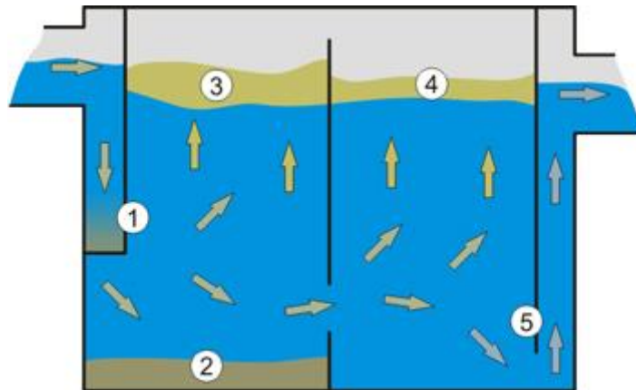
Рисунок 3 - Принцип работы
