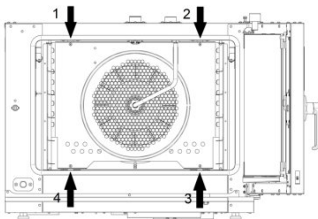
Рис. 7 Снятие перегородки
