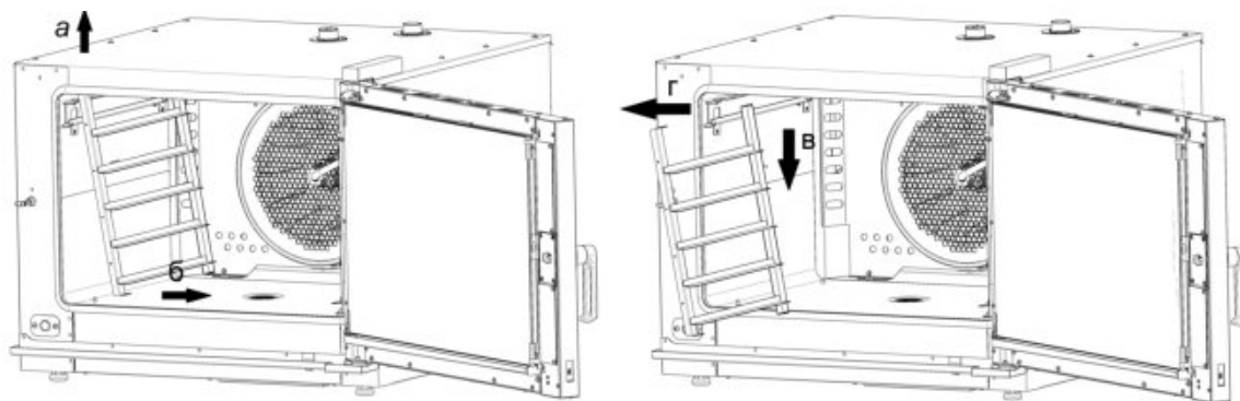
Рис. 6 Снятие направляющих
