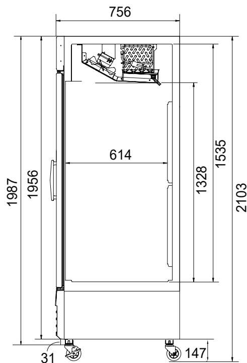
ВИД СБОКУ
