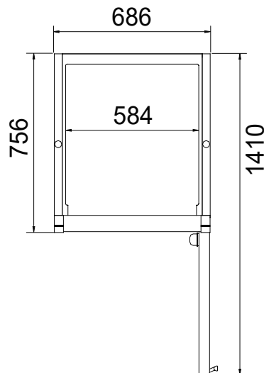
ВИД СВЕРХУ
