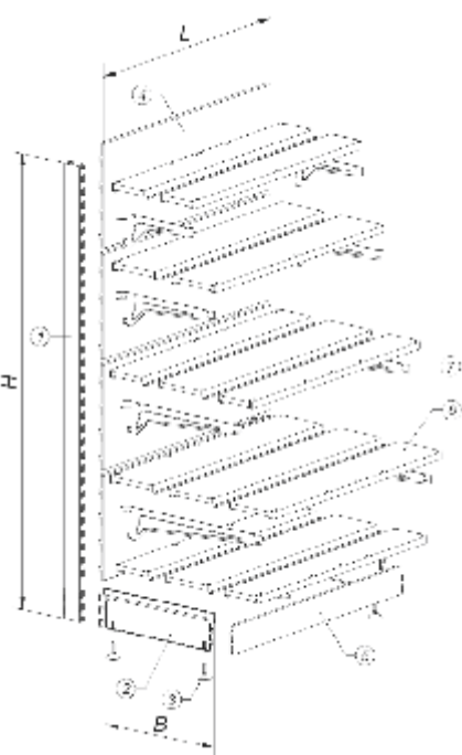
Основные элементы стеллажа «Эконом»
