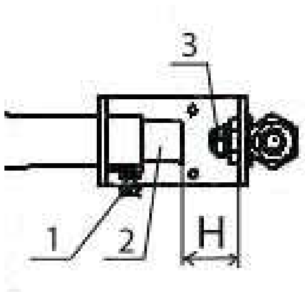
Рис. 10 Горелка духовки
