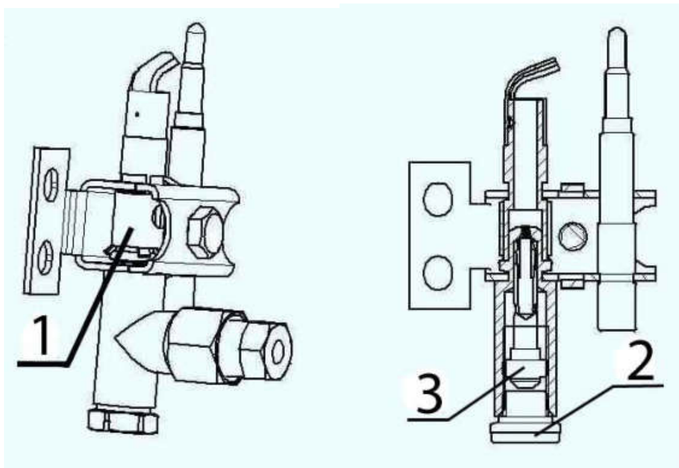
Рис. 11 Запальная горелка стола (пилот)
