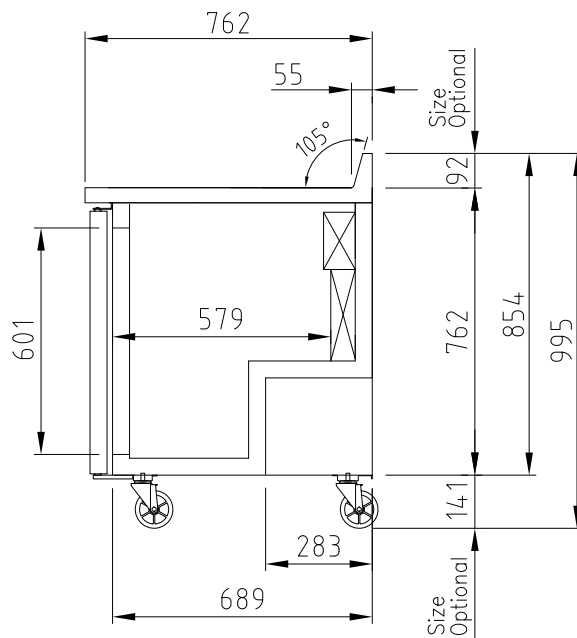
ВИД СБОКУ
