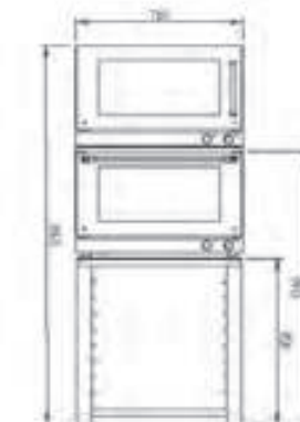
RXL 604 PLUS RX 604 PLUS SOPORTE RX 60_40 KIT SUPERPOSICIÓN SERIE RX 60_40
