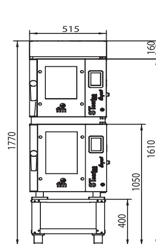
CAMPANA ST COMPACT ST-C411 V5 ST-C611 V5 KIT SUPERPOSICIÓN ST-C400
