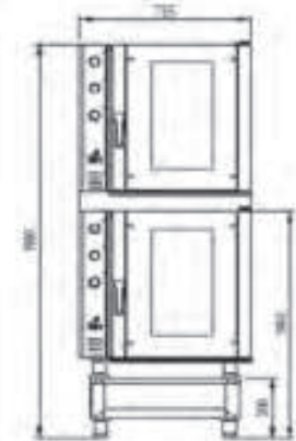
RXB 606 RXB 606 SOPORTE RXB300 300 KIT SUPERPOSICIÓN SERIE RXB
