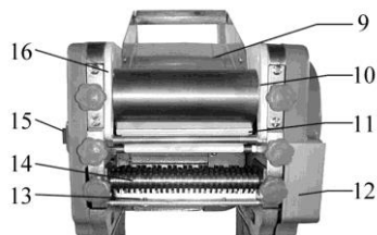
Рис 2: Вид спереди
