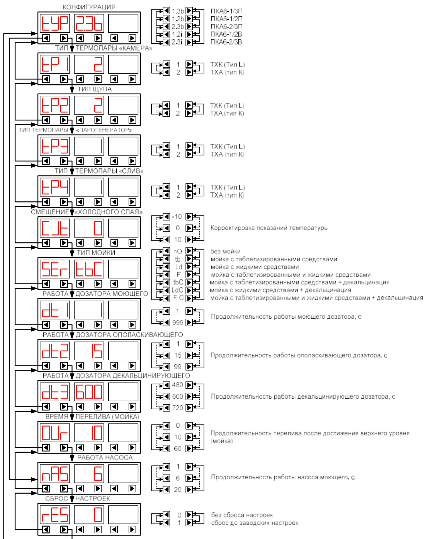
Рис.9. Настройка контроллера
