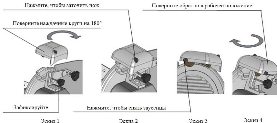
Рис.8 - заточка ножа
