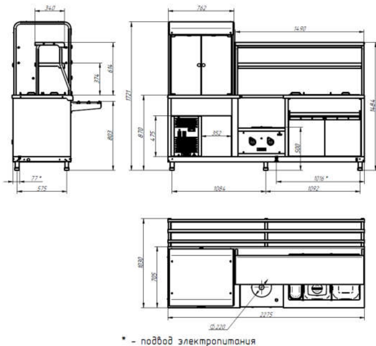
Рис. 1 Общий вид прилавка-витрины холодильной мармита ПВХМ-70КМУ правый
