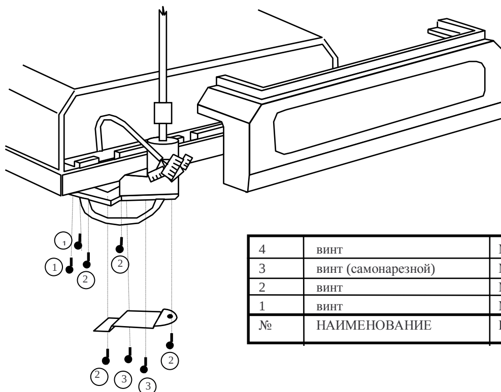
Рис. 3. УСТАНОВКА СТОЙКИ ДИСПЛЕЯ
