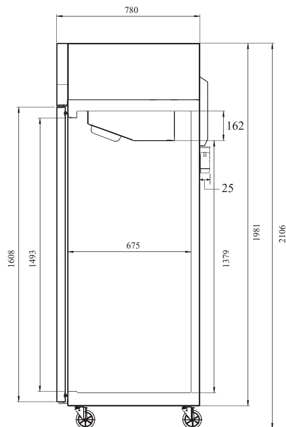
ВИД СБОКУ
