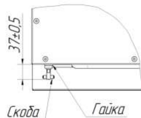
Рис. 8. Регулировка замкового устройства
