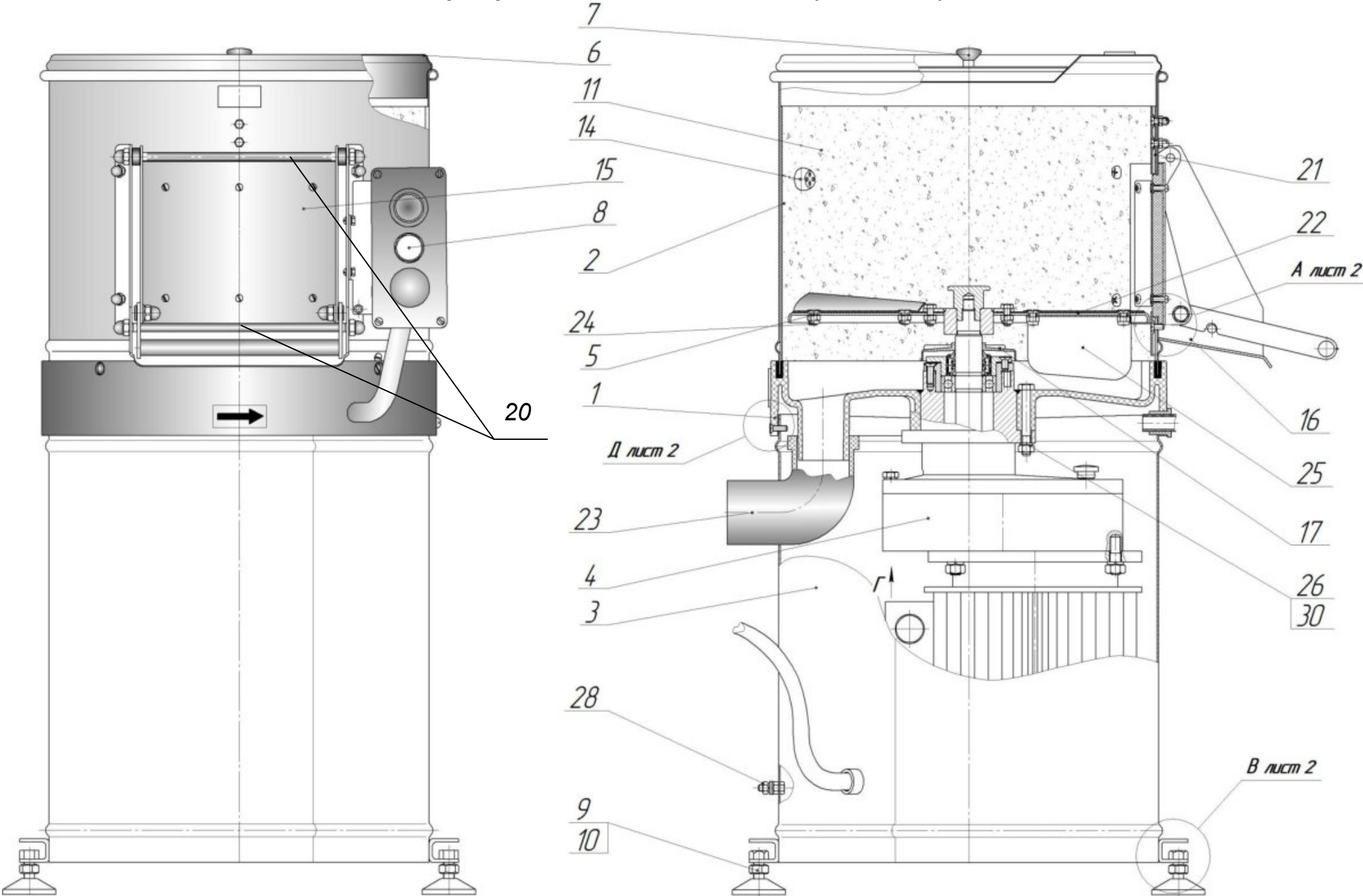
Машина картофелеочистительная К-300 (без литья), лист 1
