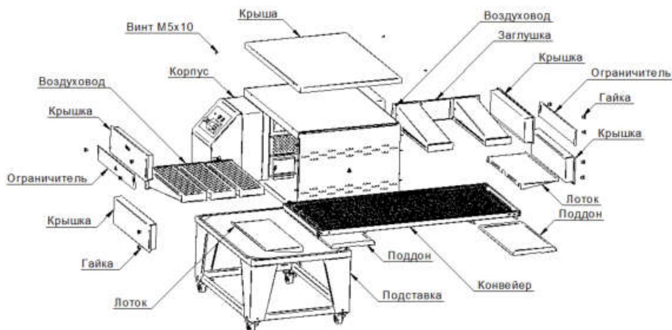
Рис. 3 - Состав изделия
