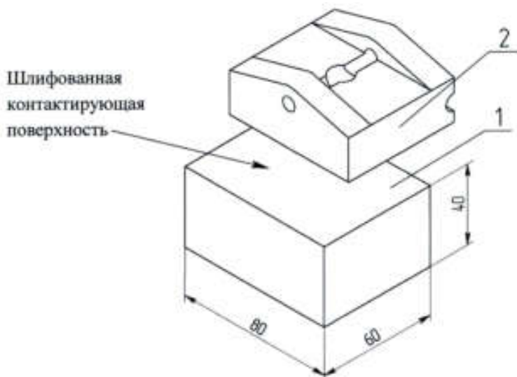
Рисунок 1 - Проверка магнита.
