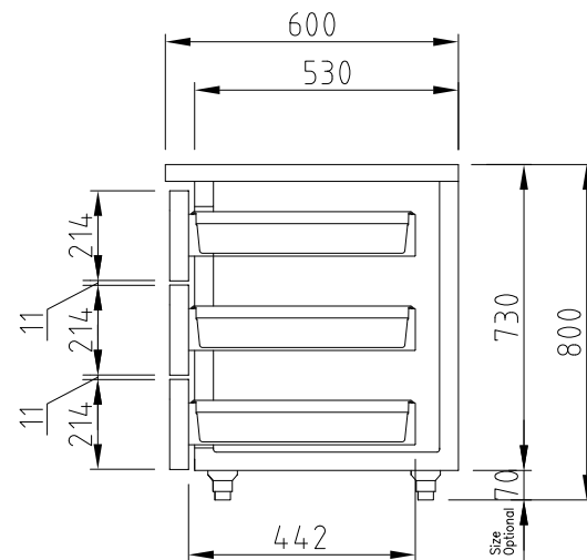
ВИД СБОКУ
