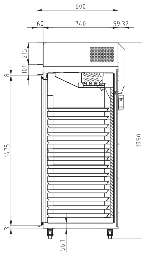
ВИД СБОКУ
