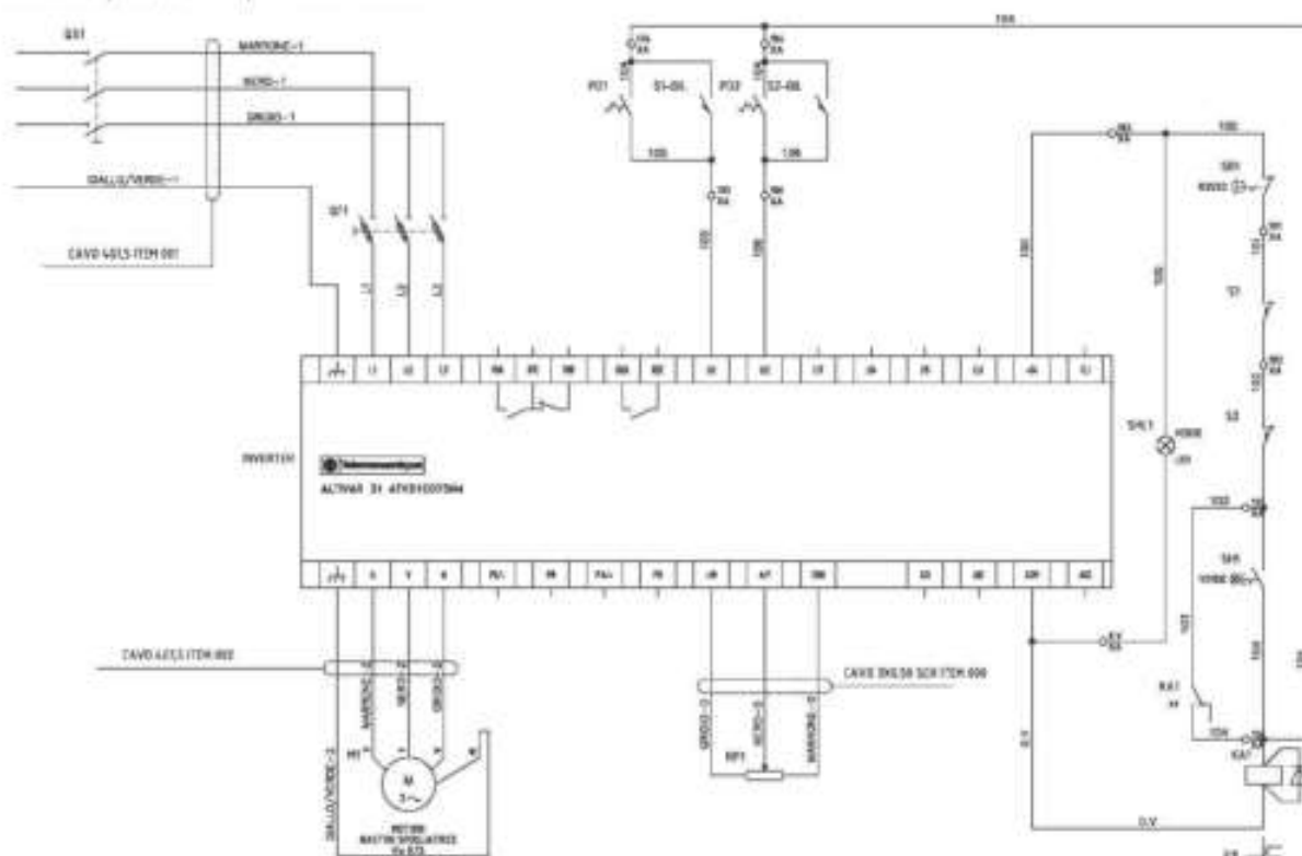
FIG. / ABB. / РИС. 19 DSF600P-DSF500P Schema elettrico / Electrical diagram / Schemas électriques / Diagramas eléctricos Elektroschaltpläne / Электрические схемы
