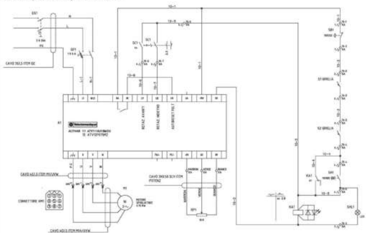
FIG. / ABB. / РИС. 17 DSB500P Schema elettrico / Electrical diagram / Schemas electriques / Diagramas eléctricos Elektroschaltpläne / Электрические схемы
