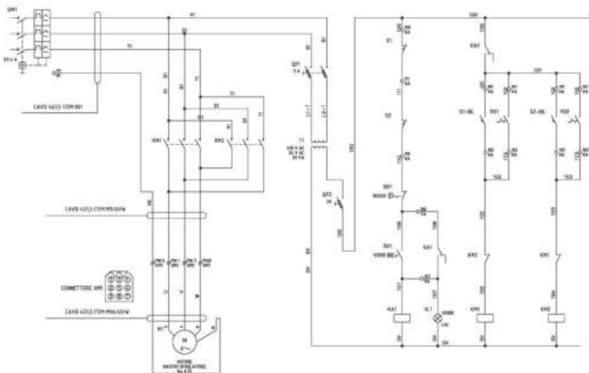
FIG. / ABB. / РИС. 18 DSB600 Schema elettrico / Electrical diagram / Schemas electriques / Diagramas eléctricos Elektroschaltpläne / Электрические схемы
