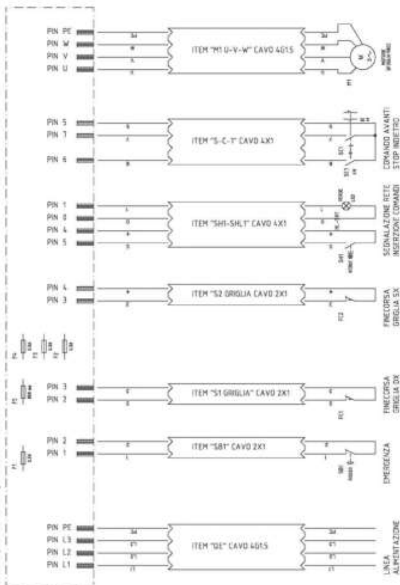
FIG. / ABB. / РИС. 16 -DSF/DSB 500 Schema elettrico / Electrical diagram / Schemas électriques / Diagramas electrónicos Elektroschaltpläne / Электронические схемы
