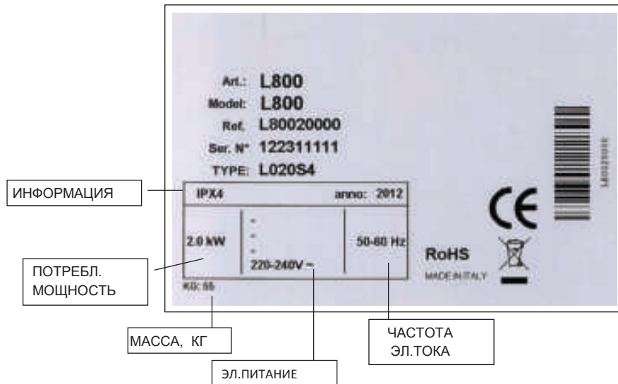
ТАБЛИЧКА ДАННЫХ
